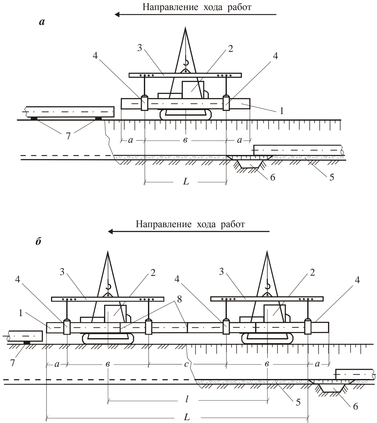
а) – при укладке одиночных труб; б) – при укладке секций 1– укладываемая труба (секция); 2 – трубоукладчики; 3 – траверса; 4 – монтажное полотно; 5 – гравийная «подушка»; 6 – прямок; 7 – лежка; 8 – межтрубные соединения
