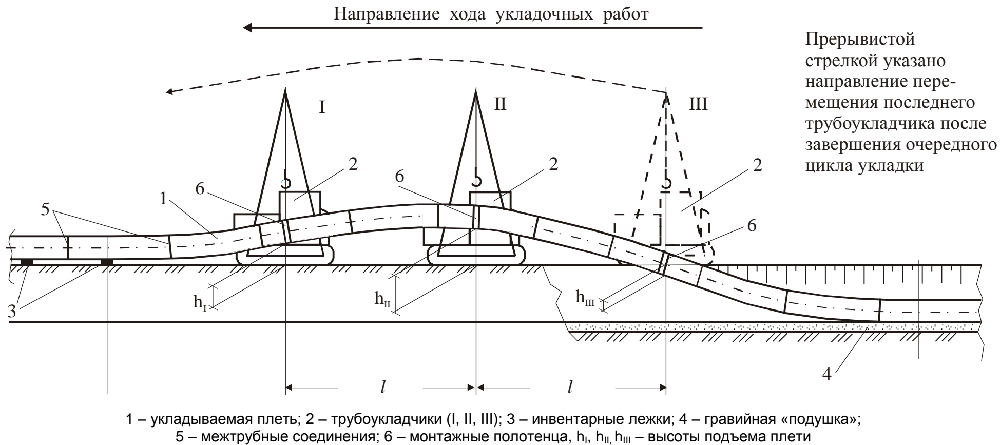
Рисунок 8 - Технологическая схема укладки длиномерных плетей при строительстве трубопроводов из стеклопластиковых труб
